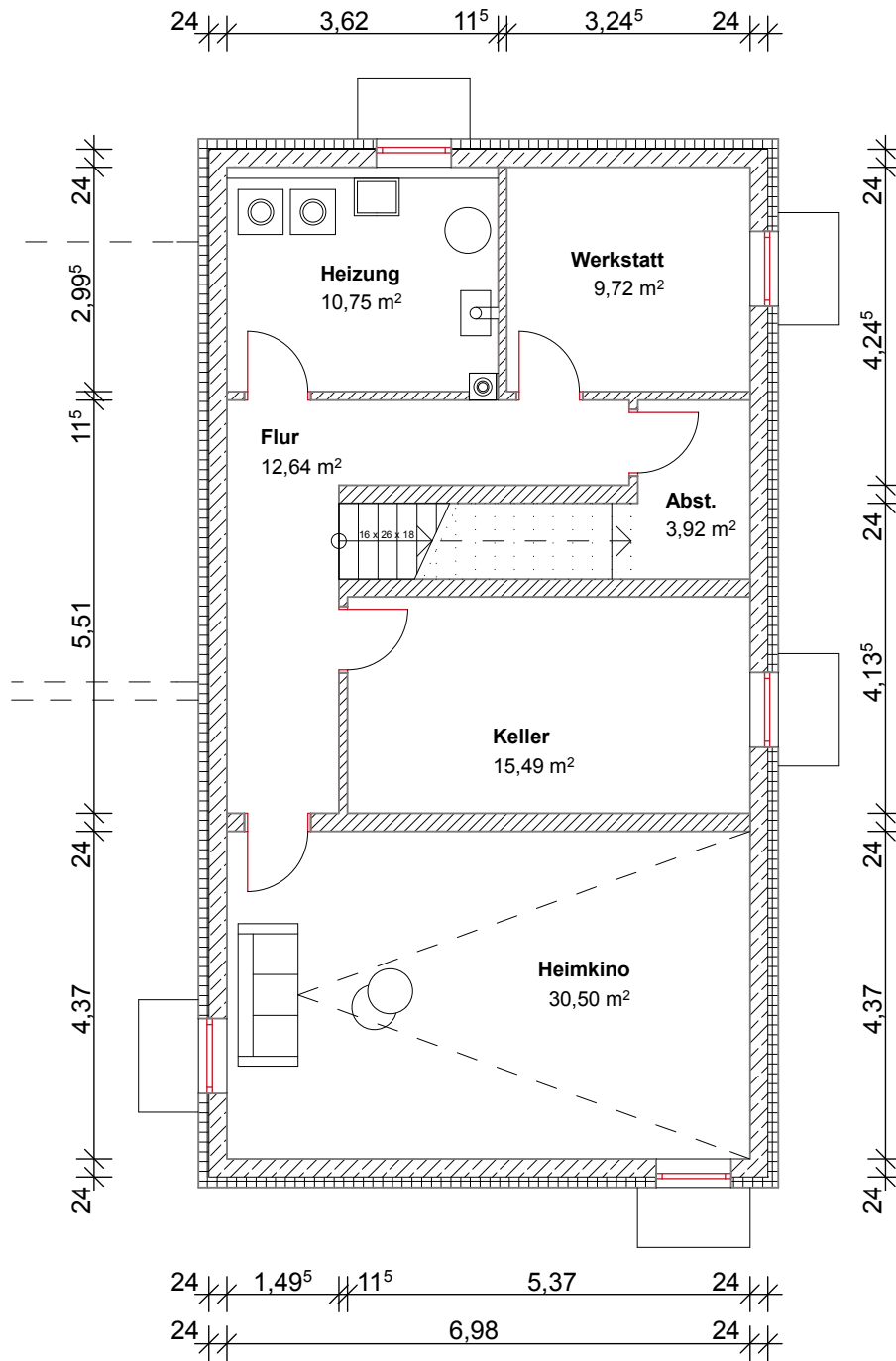
Grundriss KG
