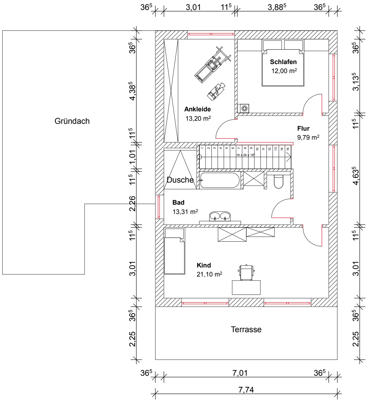
Grundriss OG
