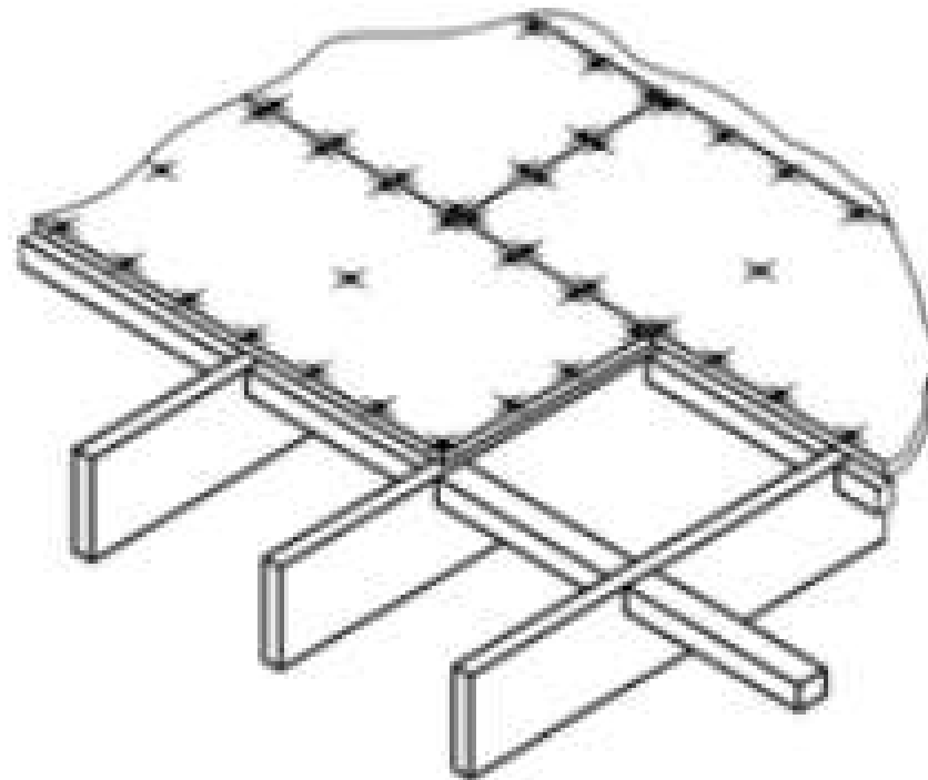
Bild 19 — Parallel besäumte tragende Dachschalung, quer zu den Balken verlegt und durch Stützleisten abgestützt
