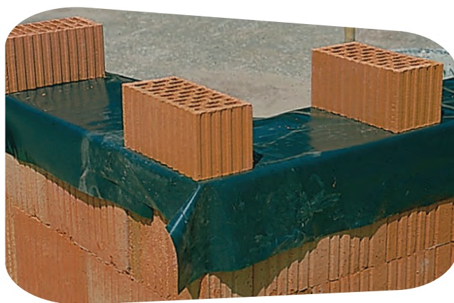
Bild 11: Schutz des Mauerwerks im Bauzustand
