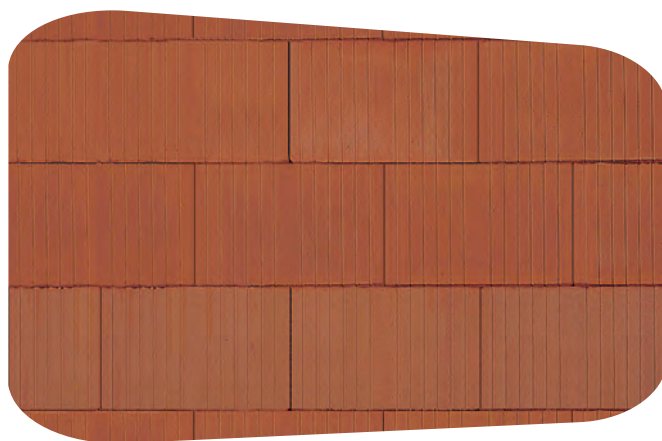
Bild 9: Normgerechtes Überbindemaß
