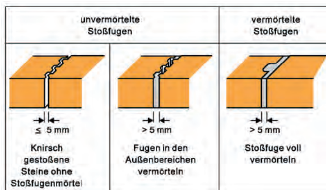
Bild 10: Stoßfugenausführung
