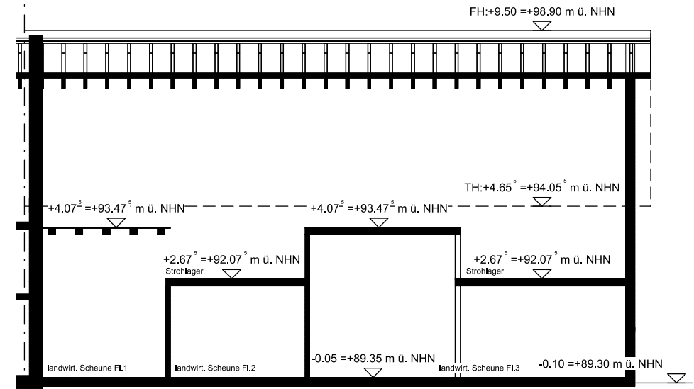
Schnitt C - C
