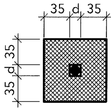
Schnitt I 1 -I 1
