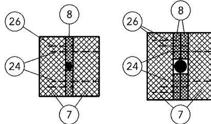
⑦ mit Zwischenlagen aus ⑧, ggf. mehrlagig
