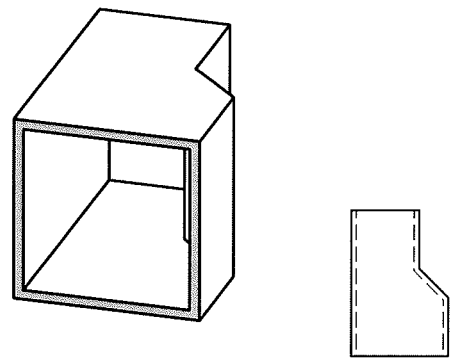
Übergang, asymmetrisch
