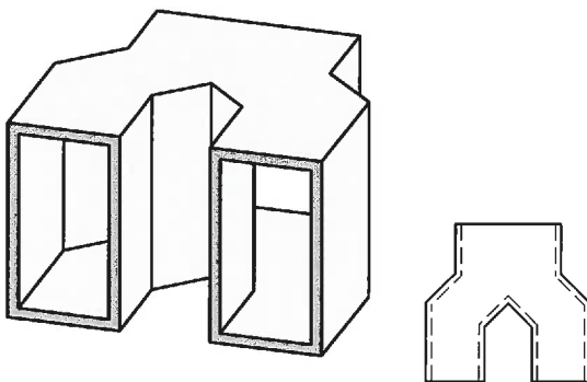
Hosenstück
