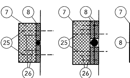
⑦ mit Zwischenlagen aus ⑧, ggf. mehrlagig
