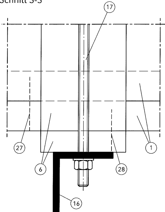
Schnitt S-S
