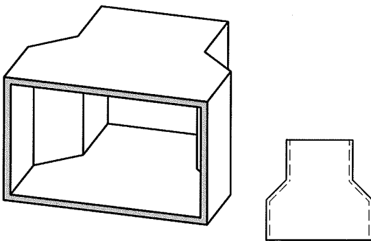
Übergang, symmetrisch
