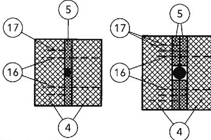
④ mit Zwischenlagen aus ⑤, ggf. mehrlagig
