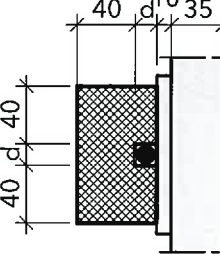
Schnitt H 2 -H 2
