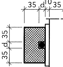
Schnitt J 1 -J 1
