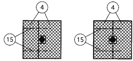
④ gefräst (einseitig oder beidseitig)
