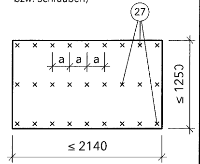
Skizze 1: Kanaldraufsicht (Anordnung der Klammern bzw. Schrauben)
