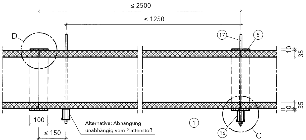
Längsschnitt
