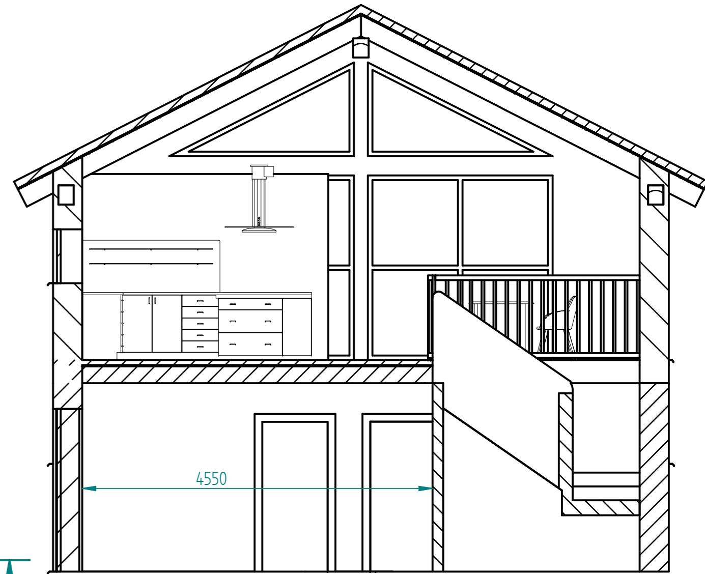
Schnitt C-C (90° gedreht)
