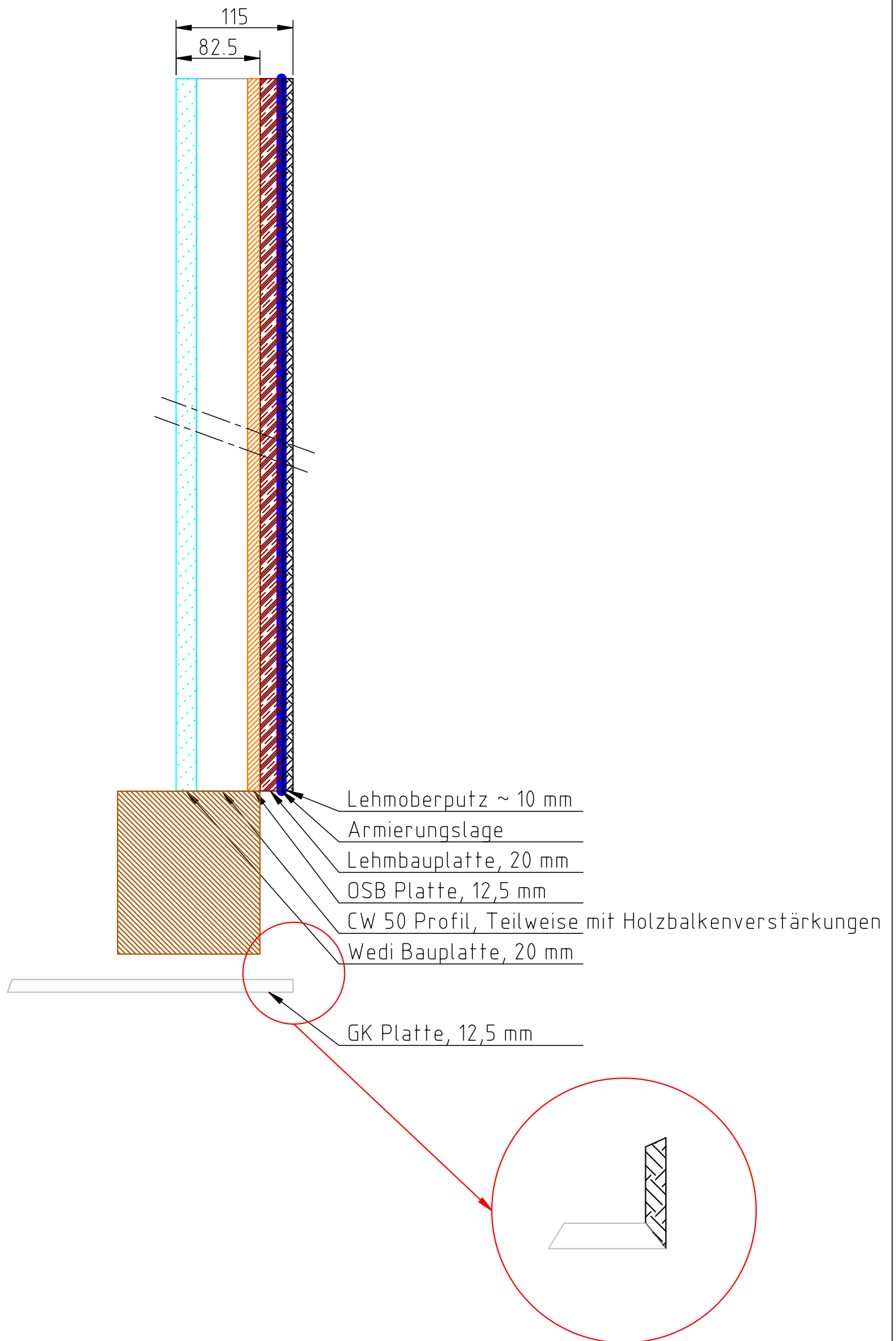
Wandaufbau, Trennwand Bad - Treppenhaus
