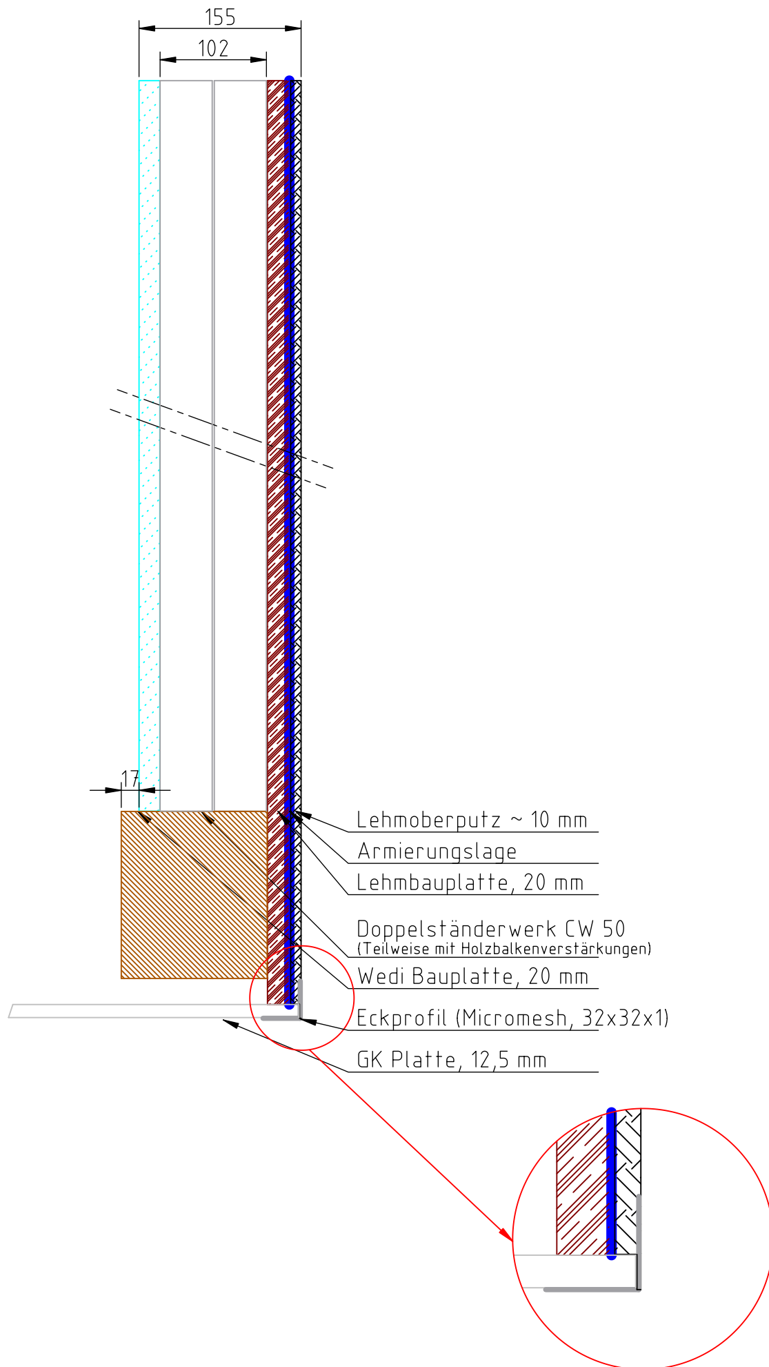
Wandaufbau, Trennwand Bad - Treppenhaus
