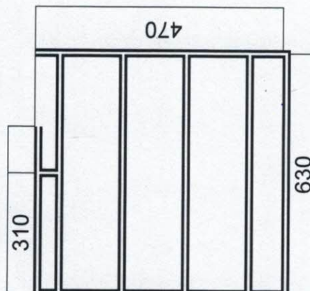
Sitzbank Seitenansicht:
